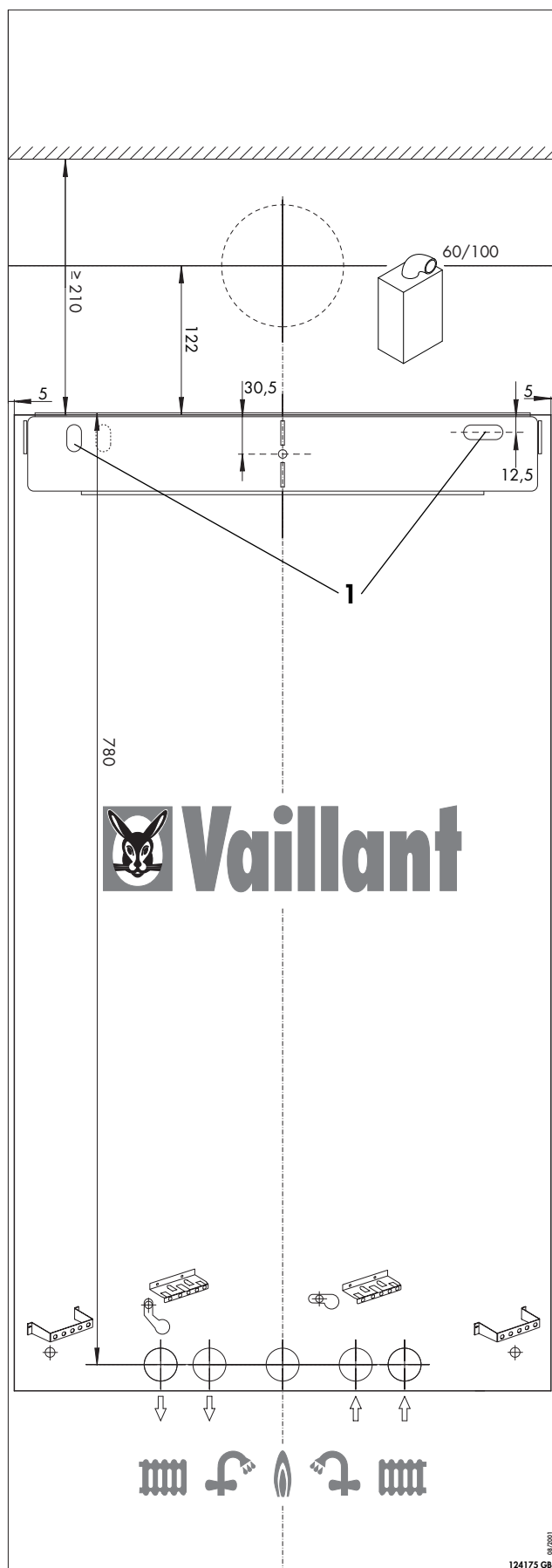
Rys. I.4: Szablony montażowe
