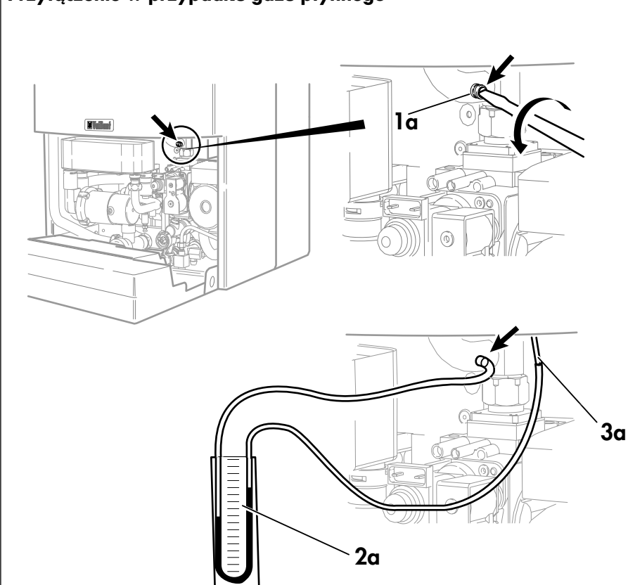
Rys. G.2: Podłączenie manometru U-rurkowego
