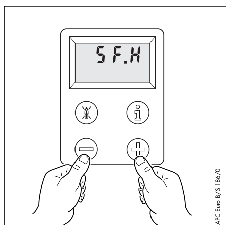
Rys. G.6: Sprawdzanie i nastawianie obciążenia częściowego w trybie ogrzewania drogą określenia natężenia przepływu gazu
