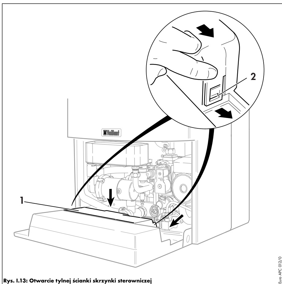
Rys. I.13: Otwarcie tylnej ścianki skrzynki sterowniczej
